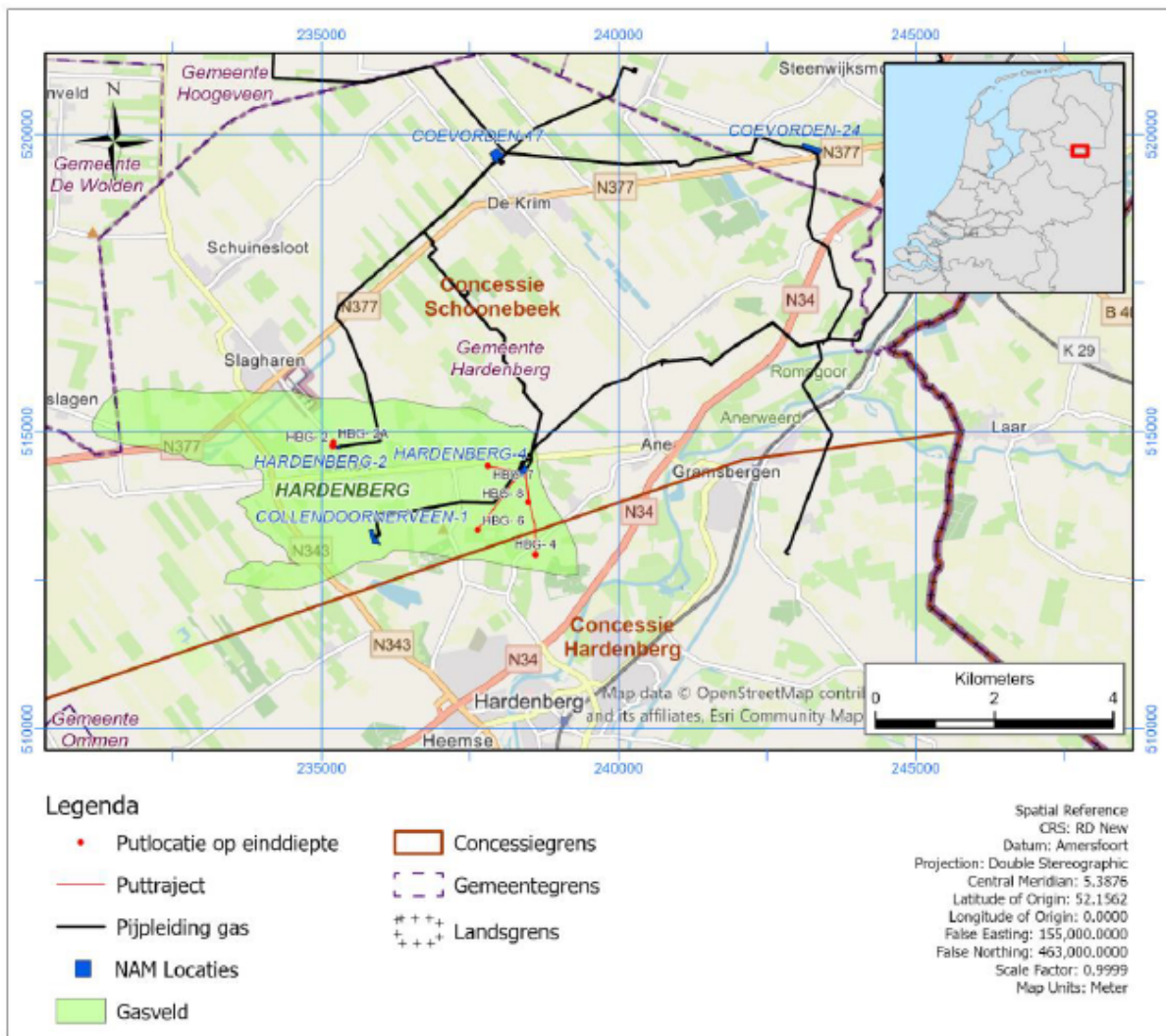
Afbeelding 1: Overzichtskarta van het gasveld Hardenberg inclusief infrastructuur.
